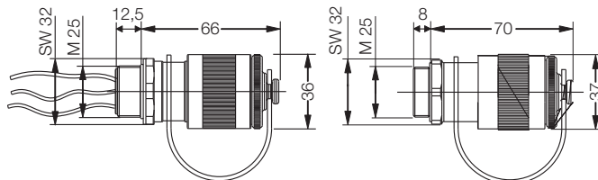
Inlet metal version: V < 2000 cm³
