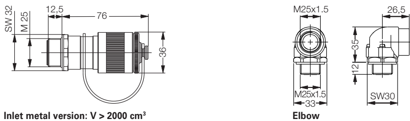
Inlet metal version: V > 2000 cm³
